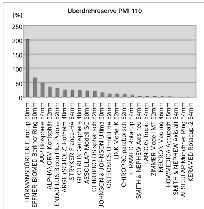
Abb. 3: Überdrehreserven der getesteten Schraubpfannen in Polymethacrylimid der Nenndichte 110 kg/m 3 .
