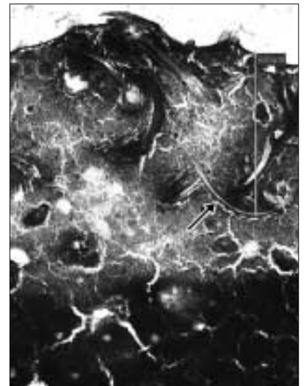
Abb. 2: Kalziumphosphatzement (Norian SRS®), PGA-PLLA-Polymervliesfasern sind im Trägermaterial verankert (→). Nach 14d Perfusionskultur. Sägeschnitt. Alcian/PAS. (Verankerungstiefe 670 µm).
